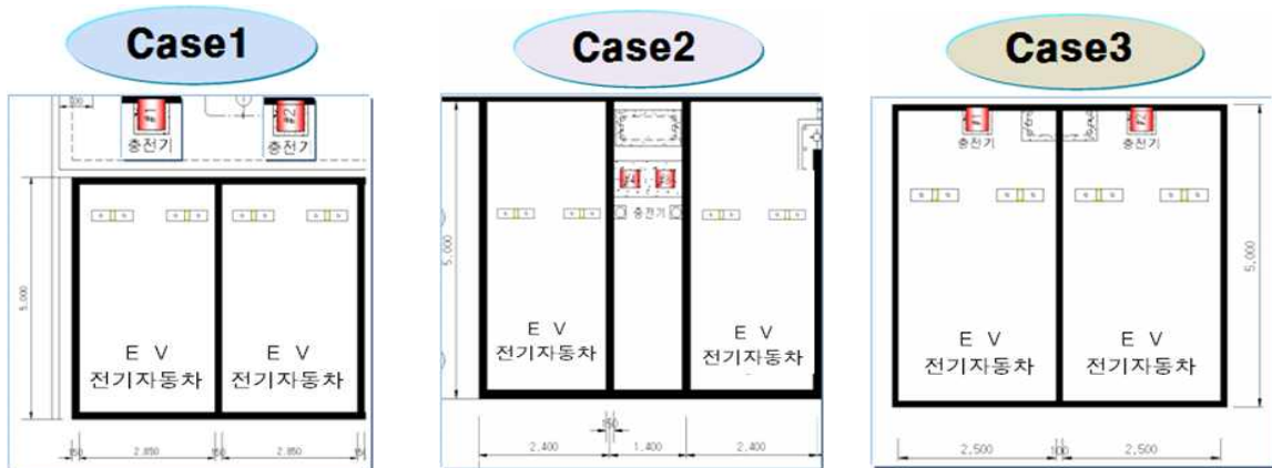
〈저공해자동차 전용 주차공간(위)과 충전기 배치사례〉
