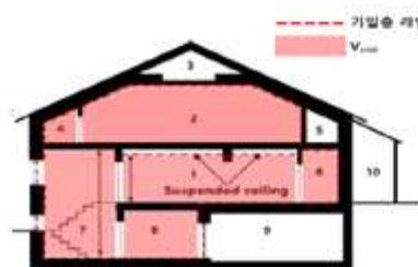
<주요 부위별 건물제적( V_{n50} ) 계산 방법>
