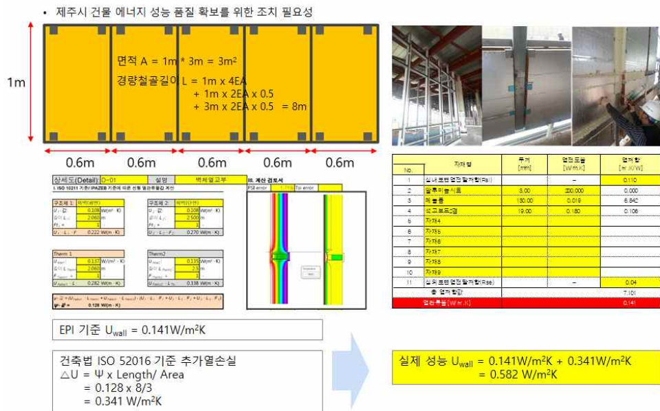
<그림> 구조체 열성능 품질 저하
